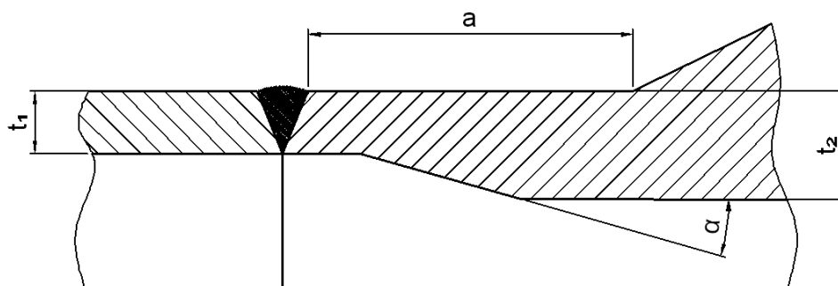
Figur 4-6. Max utvändig fasvinkel direkt vid svetsfog
