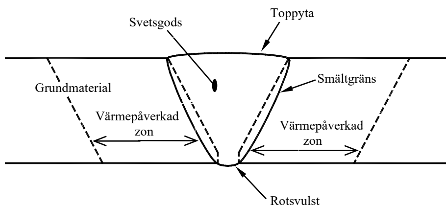
Figur 3-1. Värmepåverkad zon, HAZ
